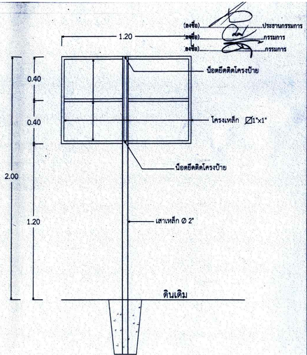
แบบแสดงรูปด้านหลังป้ายโครงการถาวร
