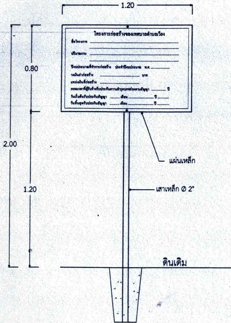
แบบแสดงรูปด้านหน้าป้ายโครงการถาวร
