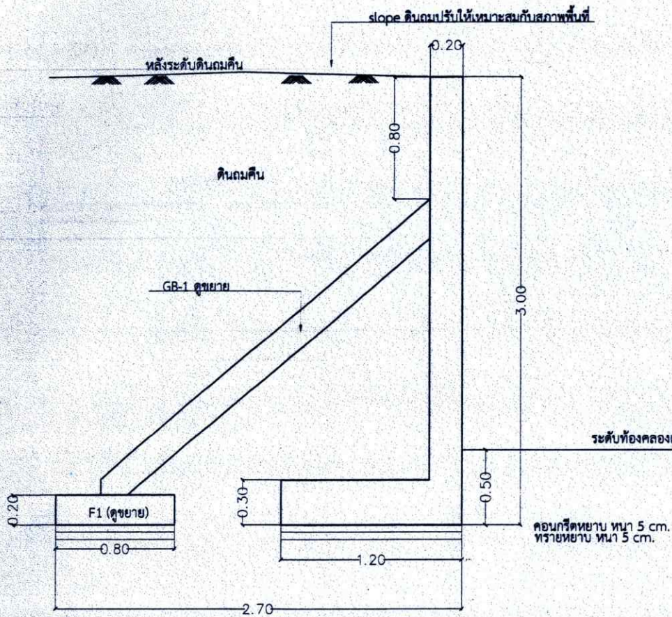
รูปตัด A - A Scale 1:25
