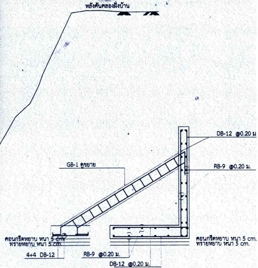
รูปตัด A - A (ขยายเหล็กเสริม) Scale
